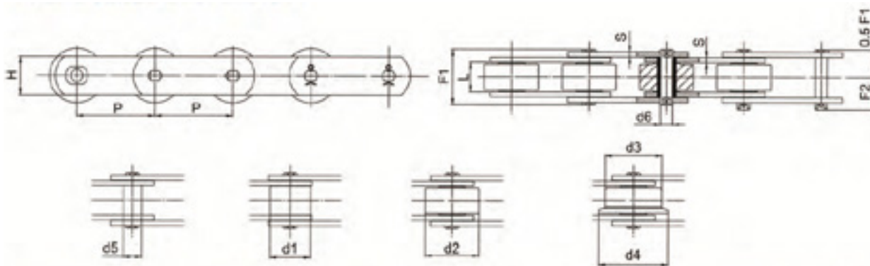
Type A (Bush type)
